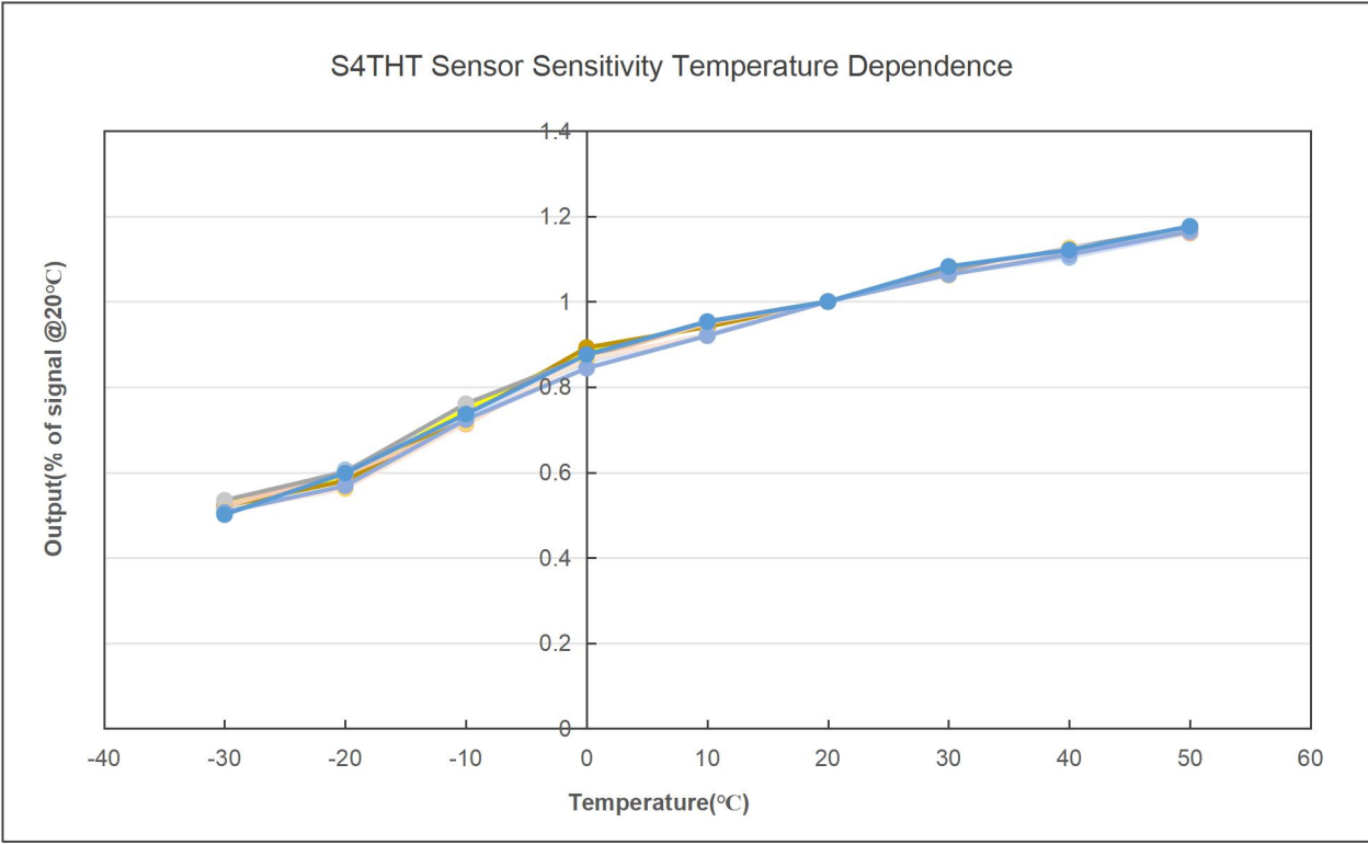
S4THT 四氢噻吩传感器灵敏度的温度依赖性曲线
