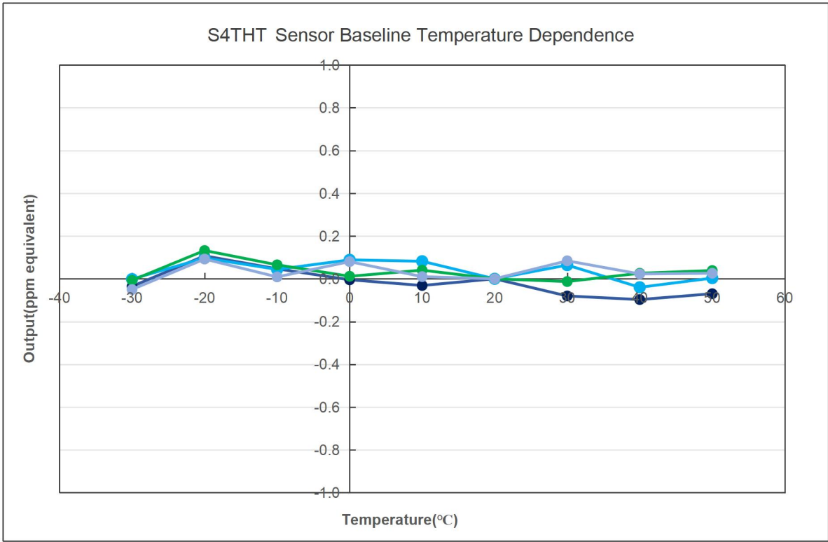
S4THT 四氢噻吩传感器基线的温度依赖性曲线
