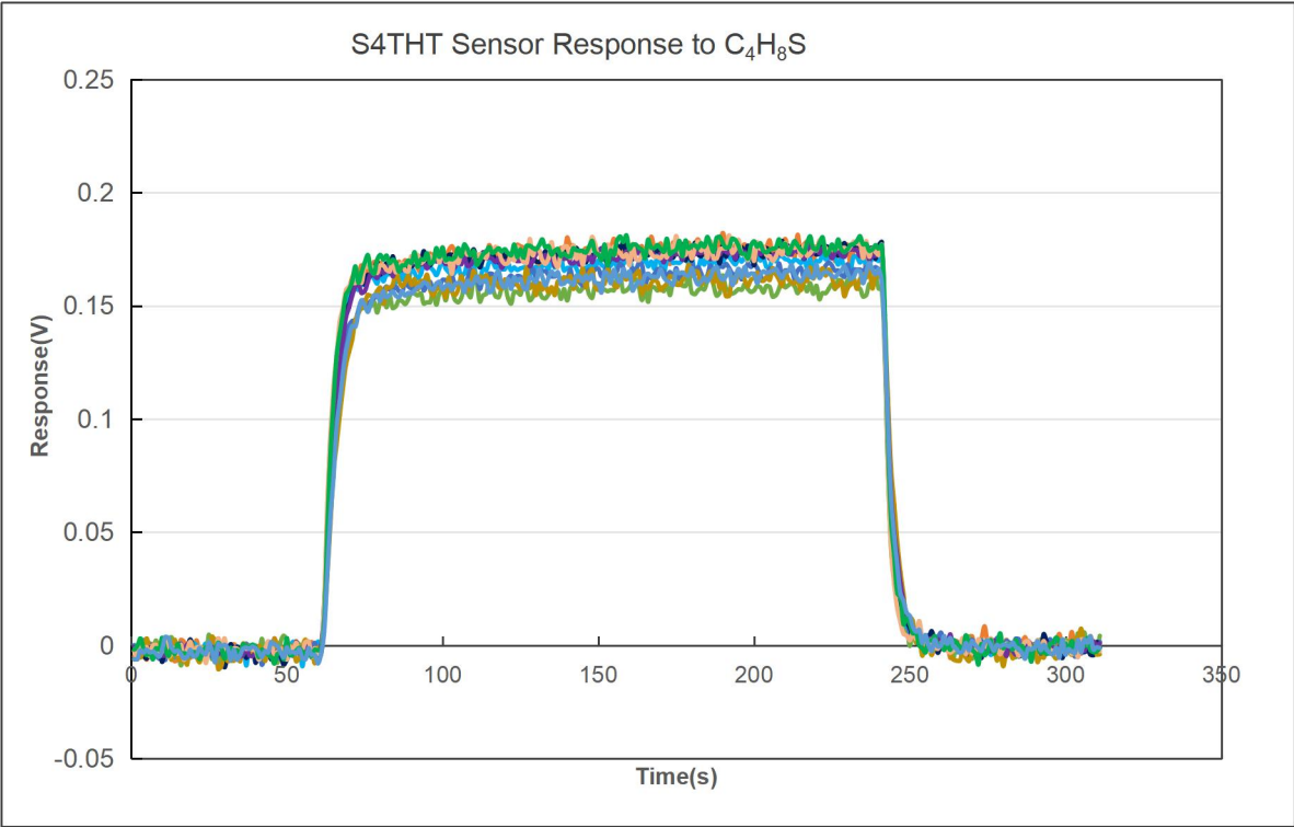
S4THT 四氢噻吩传感器的响应恢复曲线
