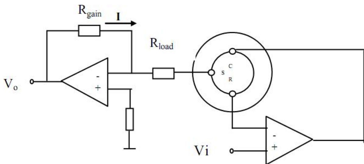
S4THT 四氢噻吩传感器的基本测试电路
