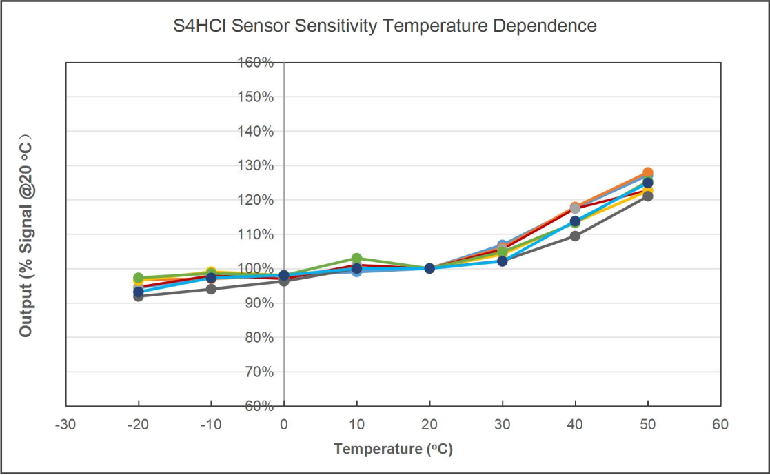
S4HCl 氯化氢传感器灵敏度的温度依赖性曲线
