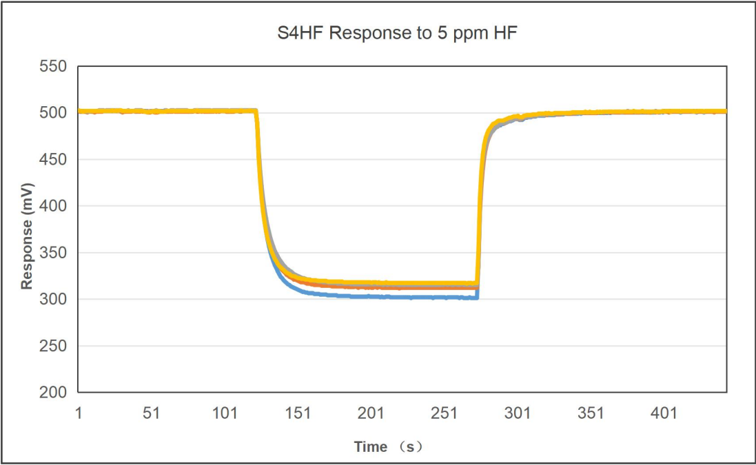
S4HF 氟化氢传感器响应恢复曲线
